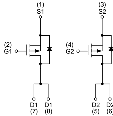
P-Channel MOSFET
